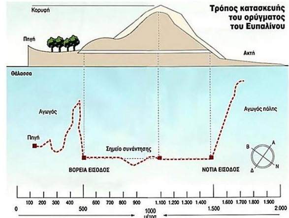
Αρχαϊκή Σάμος Το Ευπαλίνο ορύγμα (μέσα του 6ου π.Χ. αι.) Έργο του μηχανικού Ευπαλίνου από τα Μέγαρα
